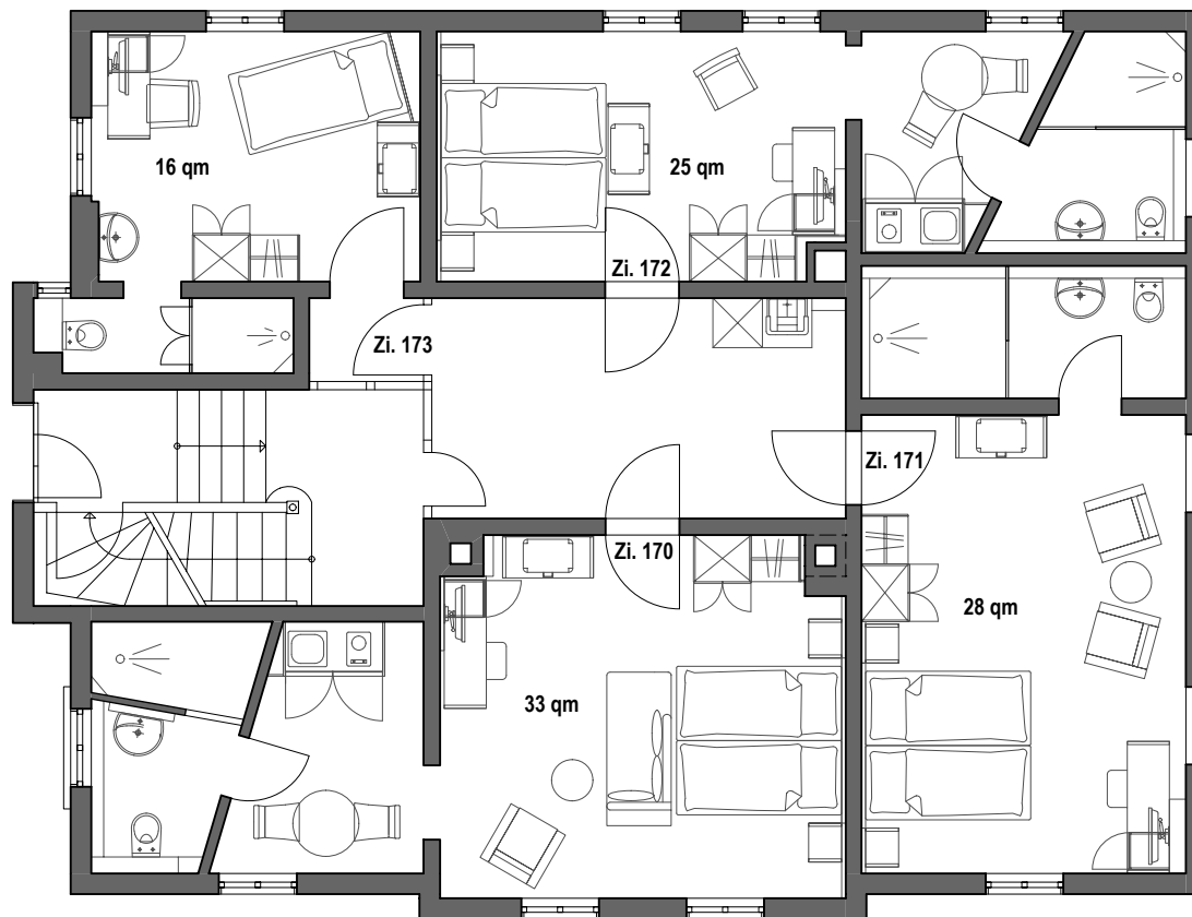
Erdgeschoss
